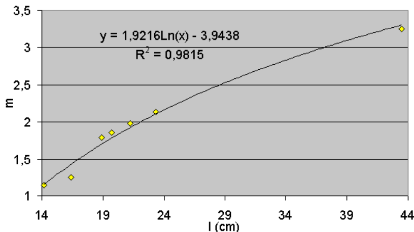
Graf 1. Ovisnost magnitude o udaljenosti na fotometru
